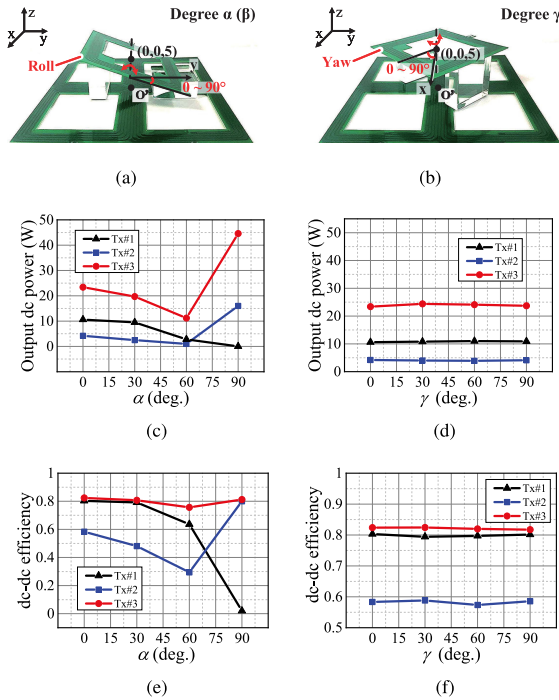
Fig. 17. Experimental results in different \alpha and \gamma angles using Tx#1, Tx#2, and Tx#3. (a) Setup ( \alpha angles). (b) Setup ( \gamma angles). (c) Output power ( \alpha angles). (d) Output power ( \gamma angles). (e) DC–DC efficiency ( \alpha angles). (f) DC–DC efficiency ( \gamma angles).
