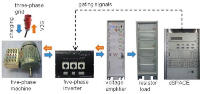
Fig. 7. Experimental rig.
